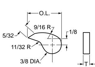
PAWL
